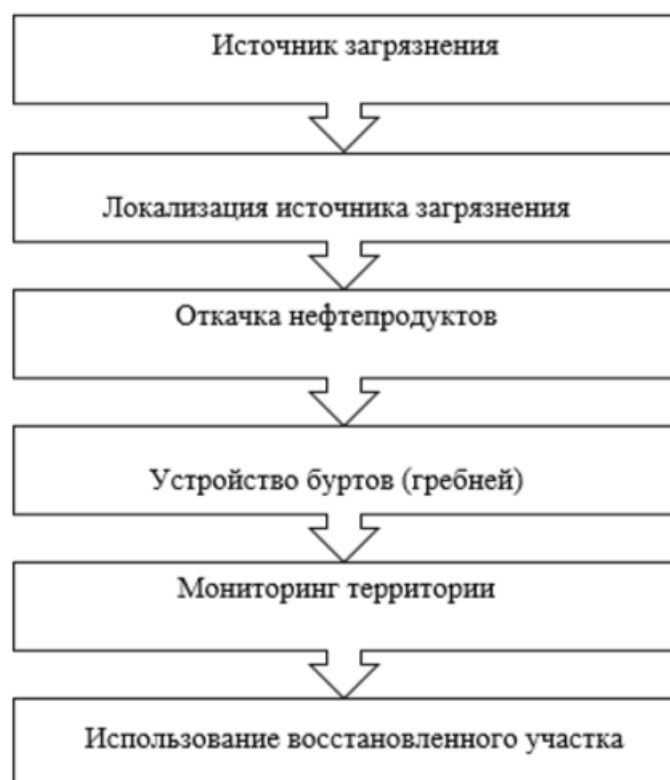
Рисунок 1. Алгоритм снижения содержания углеводородов в загрязненных торфяных грунтах
