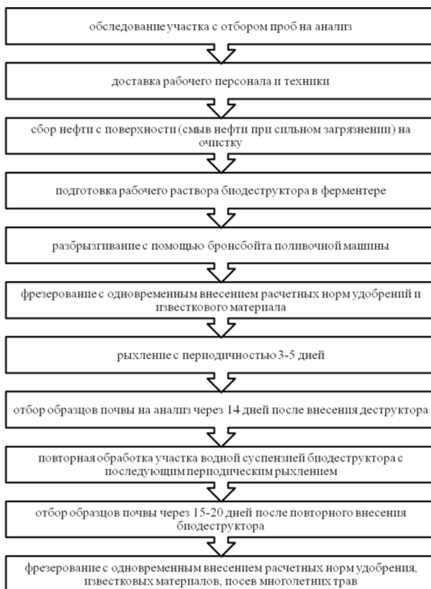
Рисунок 3. Алгоритм существующей технологии рекультивации нефтезагрязненных земель
